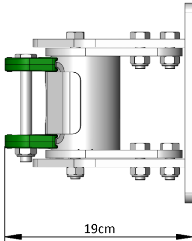
Montage / Mounting mini
